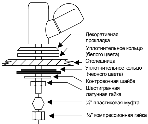
Рис.1 Установка дополнительного крана на мойку
